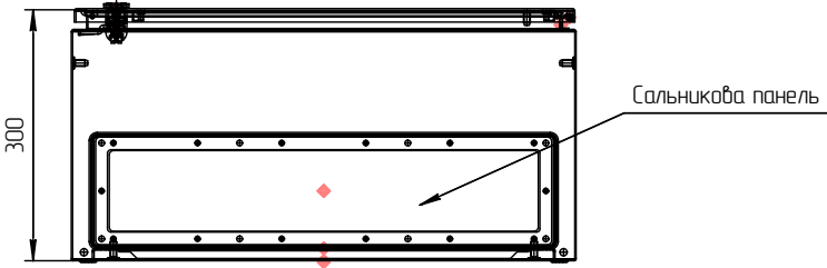
Вид знизу
